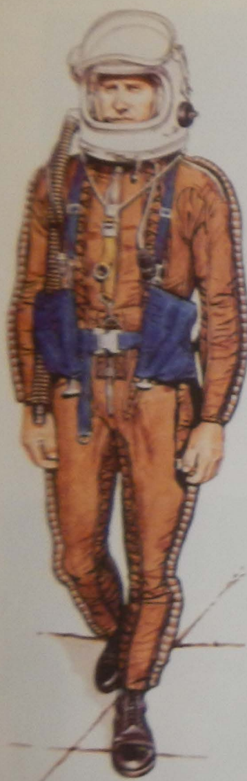
VKK-3M-G-pak en GSh-4-helm voor vliegtuigen zonder drukcabines
