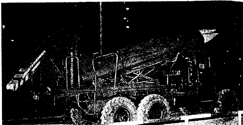
Herbevoorravingsvoertuig ZIL-131
